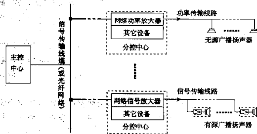
图3 有源终端和无源终端相结合的方式
